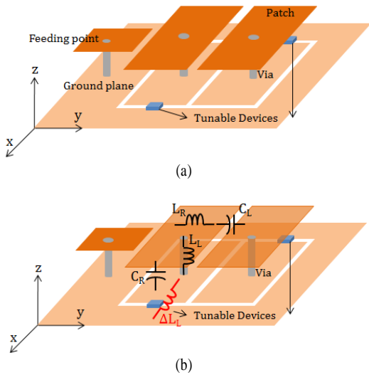
그림 2. (a) 제안된 안테나의 구조, (b) 제안된 안테나의 등가회로 모델 Fig. 2. (a) Geometry of the proposed antenna, (b) Equivalent circuit model of the proposed antenna.
