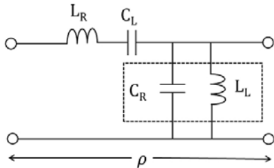
그림 1. CRLH 전송 선로의 등가회로 Fig. 1. Equivalent circuit of the CRLH transmission line.
