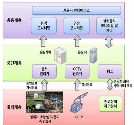
그림 1. UGMS 구조 Fig 1. UGMS Structure
