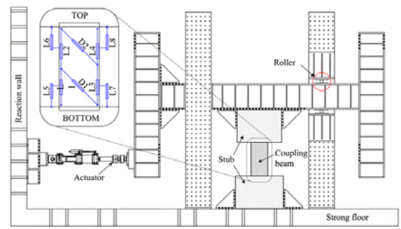
Fig. 3 Test setup
