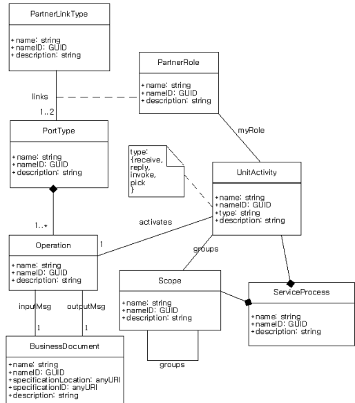
그림 5. WS-BPEL 메타데이터 온톨로지[25]
