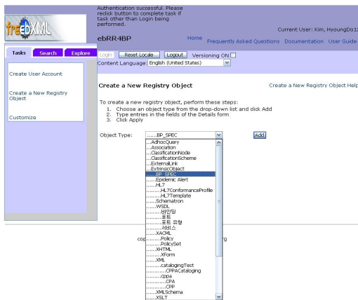
그림 10. ebRR4BP 웹 인터페이스 구성
