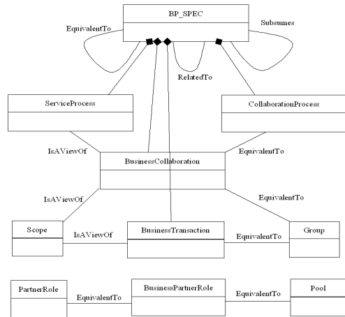
그림 6. 상호연관관계 메타데이터의 구성[25]
