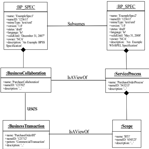
그림 7. 상호연관관계 메타데이터 사례
