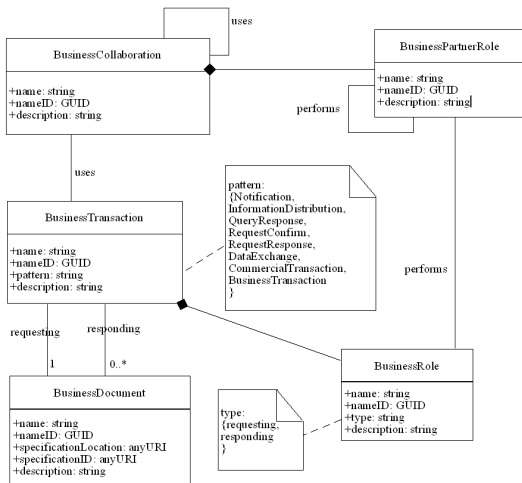
그림 4. ebXML BPSS 메타데이터 온톨로지[25]
