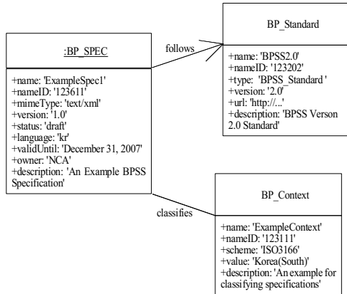
그림 3. 공통 메타데이터 사례
