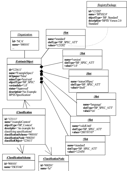
그림 9. 공통 메타데이터의 변환 결과
