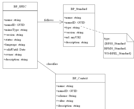
그림 2. 공통 메타데이터 온톨로지[25]
