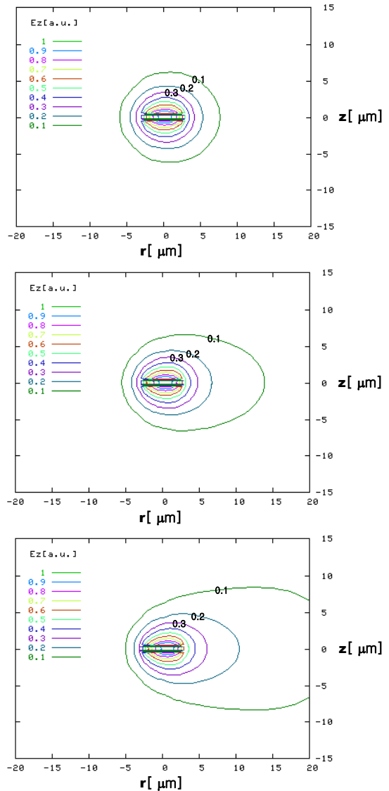
그림 6. 이중 금속선 곡선형 도파로의 R에 따른 전장 E_z 의 분포. ( D = 0.5 \text{ μm} , n_2 = 1.46 )
