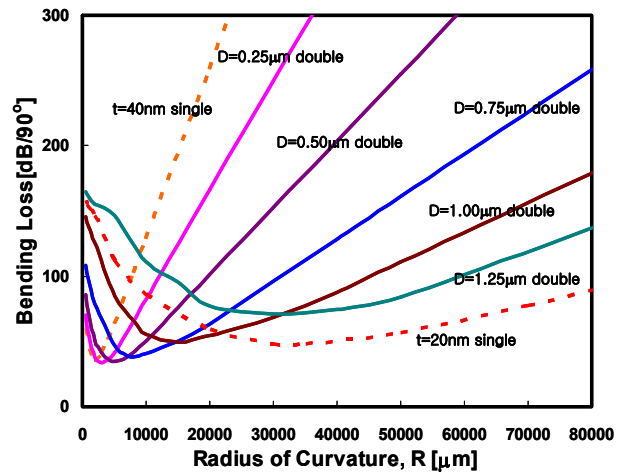
그림 8. 이중 금속선 곡선형 도파로의 최적반경과 손실. ( n_2 = 1.46 ).
