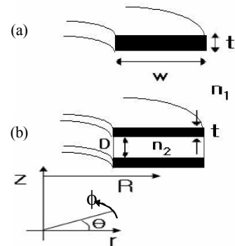
그림 1. 두 가지 형태의 곡선형 도파로 구조.
